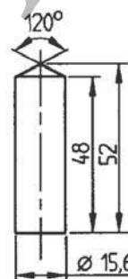
Fig. 3: Cylindrisk bronskolv, mått i mm.
