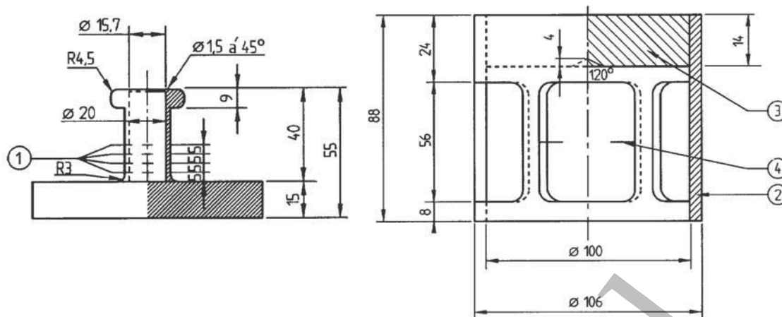
Fig. 2: Klockformig belastningstyngd, vikt 2 220 g, upphängningsbar på bronskolven, mått i mm.
