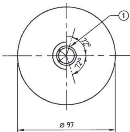
Fig. 1: Ihålig bronscylinder, tillsluten i ena änden, horisontal- och vertikalprojektion, mått i mm.
