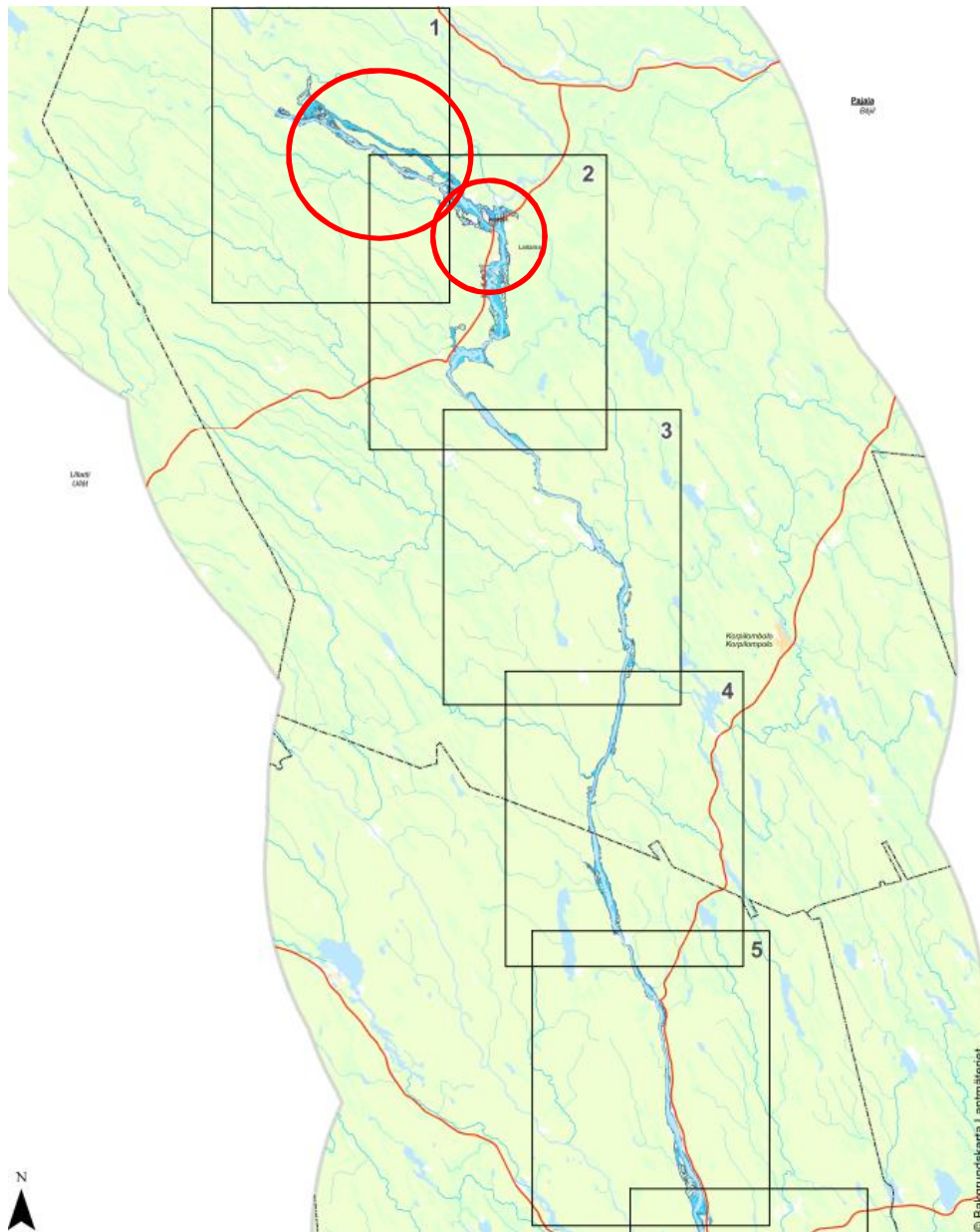
Figur 1 Område i Kalixälven där extra branch dragits samt där en 2D-modell krävs för att korrekt beskriva området.
