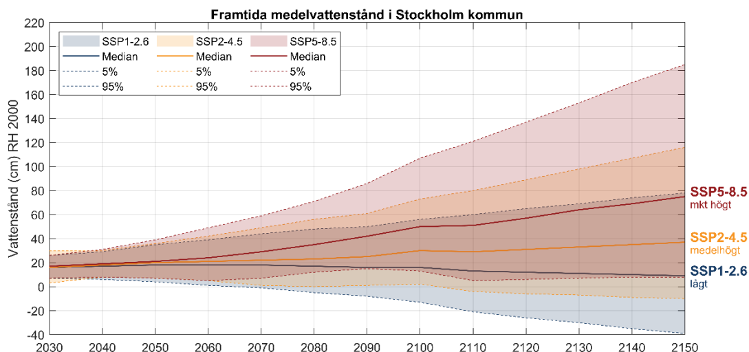
Figur 5. Utveckling av framtida medelvattenstånd i Stockholms kommun under tre olika scenarier, lågt (SSP1-2,6), medelhögt (SSP2-4,5) och mycket högt (SSP5-8,5). Medianvärden visas som heldragna linjer och de skuggade fälten täcker de mycket sannolika intervallen (5:e till 95:e percentil).
