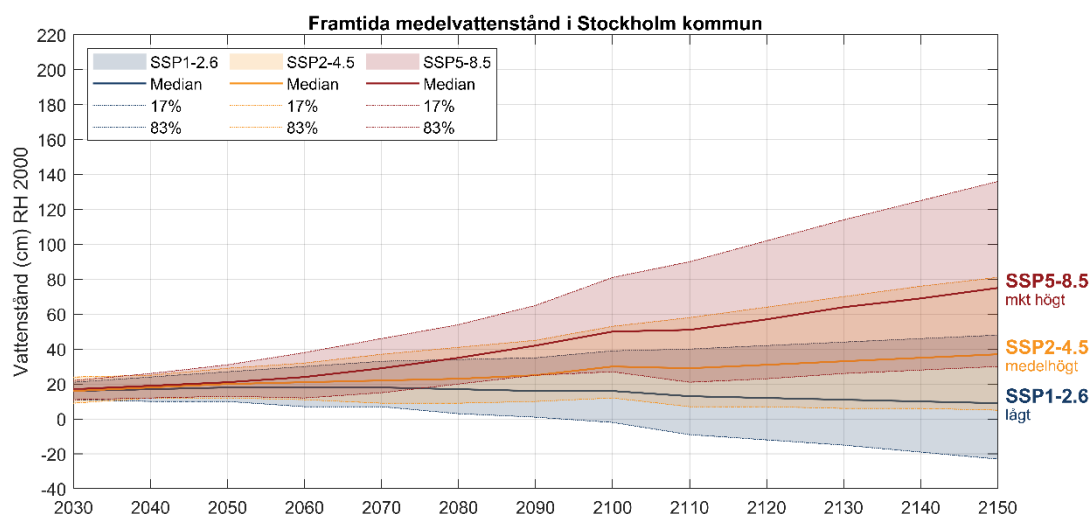
Figur 4. Utveckling av framtida medelvattenstånd i Stockholms kommun under tre olika scenarier, lågt (SSP1-2,6), medelhögt (SSP2-4,5) och mycket högt (SSP5-8,5). Medianvärden visas som heldragna linjer och de skuggade fälten täcker de sannolika intervallen (17:e till 83:e percentil).
