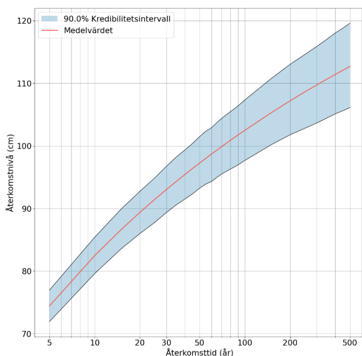
Figur 3. Återkomstnivå relativt medelvattenståndet (cm) mot återkomsttid (år) för den centrala positionen Stockholm, beräknat med den Bayesianska modellen. Medelvärde visas med röd linje och kredibilitetsintervall (Bayesiansk motsvarighet till konfidensintervall) med blå skuggning.
