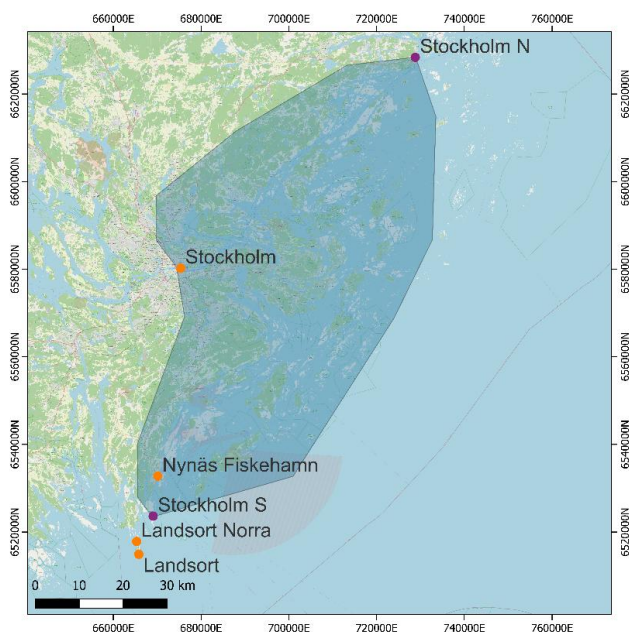
Figur 1. Geografiskt avgränsat område vid Stockholm specificerat av MSB. I kartan visas även mätstationerna vid Stockholm, Nynäs Fiskehamn, Landsort Norra och Landsort (orange) samt de positioner för vilka återkomstnivåer har beräknats med den Bayesianska modellen (orange och lila). Bakgrundskarta: OpenStreetMap.
