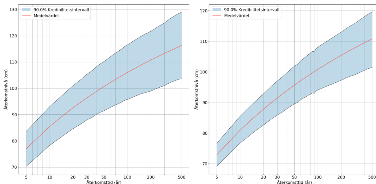
Figur 3. Återkomstnivå relativt medelvattenståndet (cm) mot återkomsttid (år) för Norrköping tätort till vänster, och för Norrköping yttre till höger, beräknat med den Bayesianska modellen. Medelvärde visas med röd linje och kredibilitetsintervall (Bayesiansk motsvarighet till konfidensintervall) med blå skuggning. Notera att y-axeln har olika skala i de båda figurerna.
