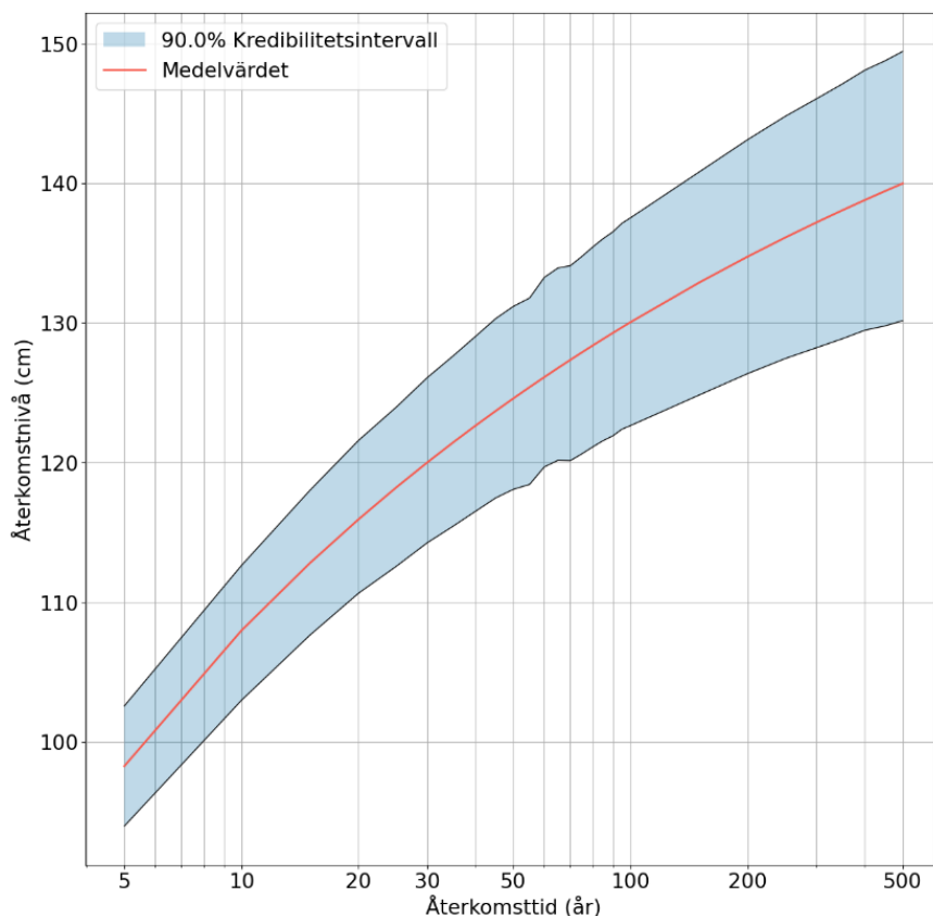
Figur 5. Återkomstnivå relativt medelvattenståndet (cm) mot återkomsttid (år) för Kristianstad, beräknat med den Bayesianska modellen. Medelvärde visas med röd linje och kredibilitetsintervall (Bayesiansk motsvarighet till konfidensintervall) med blå skuggning.
