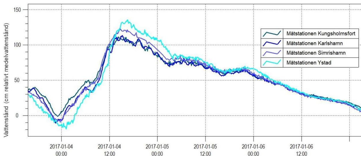
Figur 4. Vattenståndet vid Kungsholmsfort, Karlshamn, Simrishamn och Ystad under januari 2017. Den generella trenden längs den här kusträckan är att vattenståndet under en högvattenhändelse blir något högre i väst än i öst, något som också återspeglas i den Bayesianska modellen.
