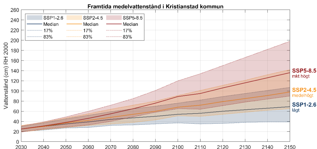
Figur 6. Utveckling av framtida medelvattenstånd i Kristianstads kommun under tre olika scenarier, lågt (SSP1-2,6), medelhögt (SSP2-4,5) och mycket högt (SSP5-8,5). Medianvärden visas som heldragna linjer och de skuggade fälten täcker de sannolika intervallen (17:e till 83:e percentil).
