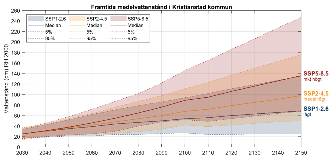
Figur 7. Utveckling av framtida medelvattenstånd i Kristianstads kommun under tre olika scenarier, lågt (SSP1-2,6), medelhögt (SSP2-4,5) och mycket högt (SSP5-8,5). Medianvärden visas som heldragna linjer och de skuggade fälten täcker de mycket sannolika intervallen (5:e till 95:e percentil).
