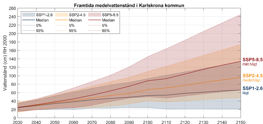
Figur 7. Utveckling av framtida medelvattenstånd i Karlskrona kommun under tre olika scenarier, lågt (SSP1-2,6), medelhögt (SSP2-4,5) och mycket högt (SSP5-8,5). Medianvärden visas som heldragna linjer och de skuggade fälten täcker de mycket sannolika intervallen (5:e till 95:e percentil).
