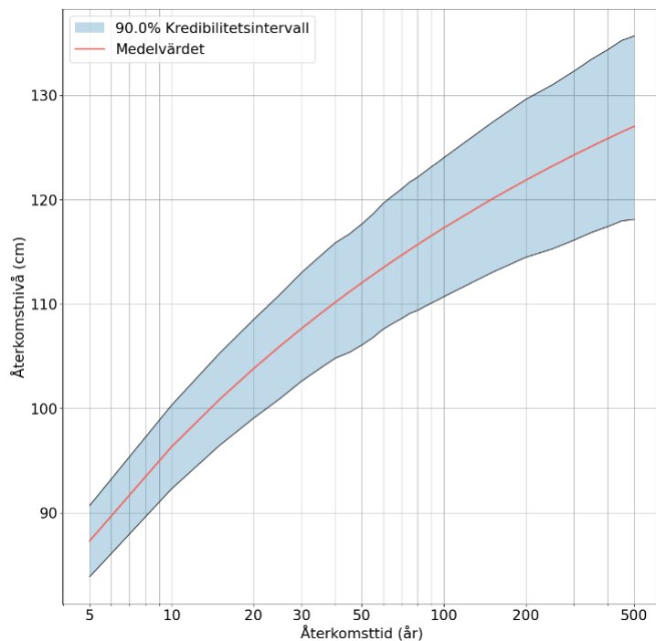
Figur 5. Återkomstnivå relativt medelvattenståndet (cm) mot återkomsttid (år) för Karlskrona, beräknat med den Bayesianska modellen. Medelvärde visas med röd linje och kredibilitetsintervall (Bayesiansk motsvarighet till konfidensintervall) med blå skuggning.
