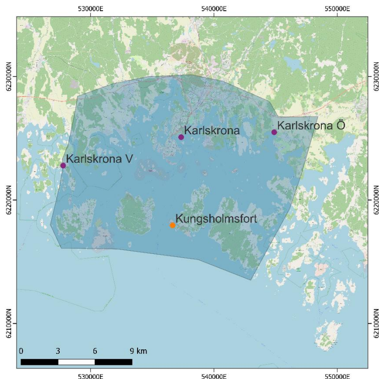
Figur 1. Geografiskt avgränsat område vid Karlskrona specificerat av MSB. I kartan visas även mätstationen vid Kungsholmsfort (orange) samt de positioner för vilka nivåer i området har beräknats med den Bayesianska modellen (lila). Bakgrundskarta: OpenStreetMap.
