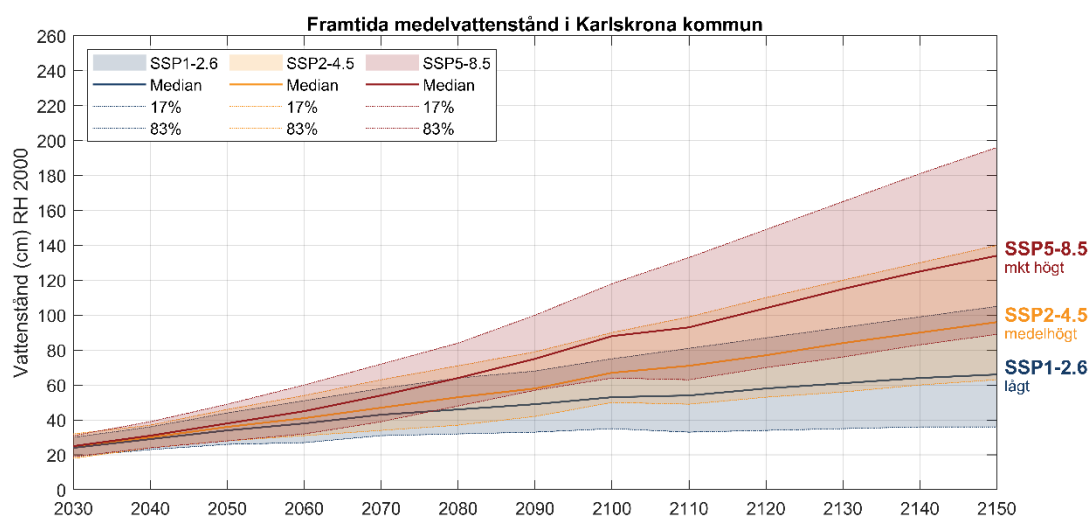
Figur 6. Utveckling av framtida medelvattenstånd i Karlskrona kommun under tre olika scenarier, lågt (SSP1-2,6), medelhögt (SSP2-4,5) och mycket högt (SSP5-8,5). Medianvärdena visas som heldragna linjer och de skuggade fälten täcker de sannolika intervallen (17:e till 83:e percentil).
