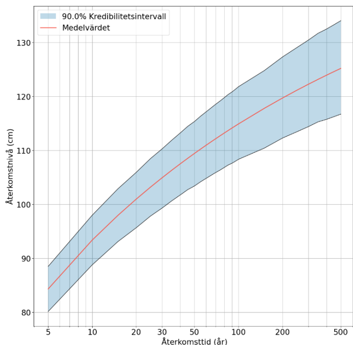
Figur 5. Återkomstnivå relativt medelvattenståndet (cm) mot återkomsttid (år) för Kalmar, beräknat med den Bayesianska modellen. Medelvärde visas med röd linje och kredibilitetsintervall (Bayesiansk motsvarighet till konfidensintervall) med blå skuggning.
