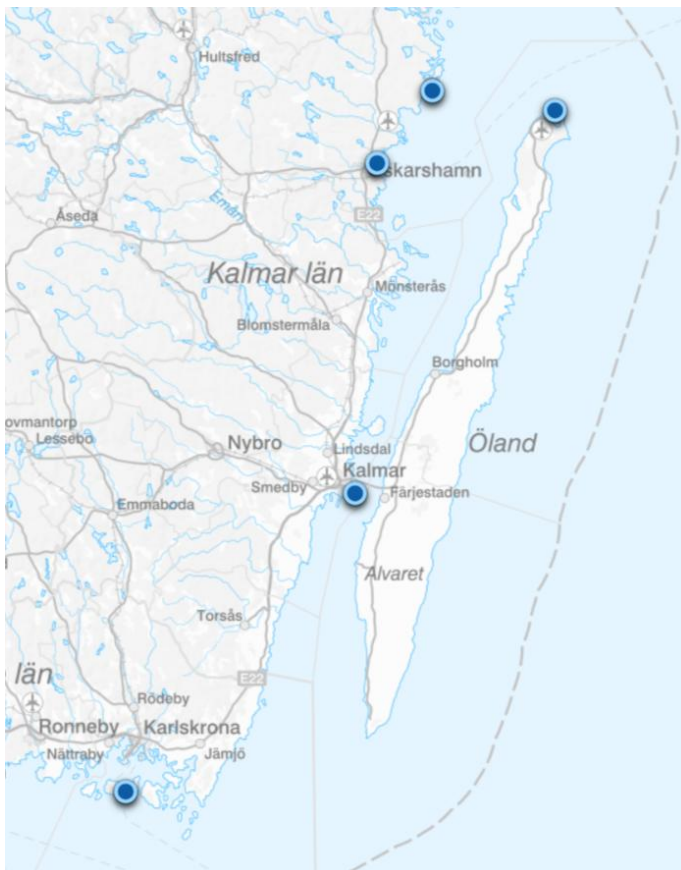
Figur 4. SMHIs och Sjöfartsverkets mätstationer längs delar av mellersta och södra Östersjökusten. Karta: SMHI.
