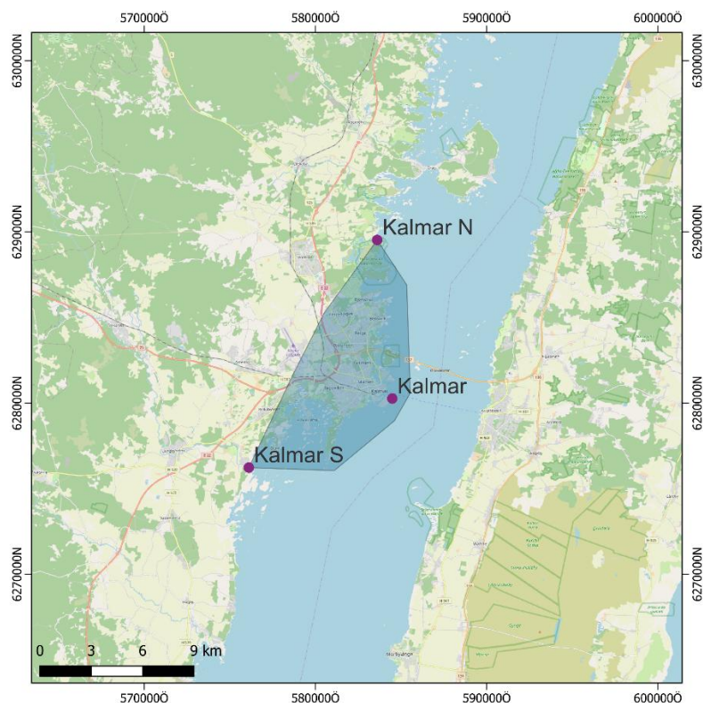
Figur 1. Geografiskt avgränsat område vid Kalmar specificerat av MSB. I kartan visas även de positioner för vilka återkomstnivåer har beräknats med den Bayesianska modellen. Bakgrundskarta: OpenStreetMap
