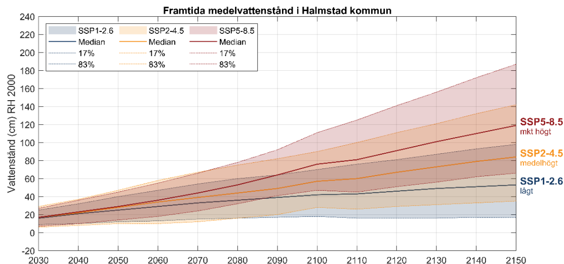
Figur 3. Utveckling av framtida medelvattenstånd i Halmstads kommun under tre olika scenarier, lågt (SSP1-2,6), medelhögt (SSP2-4,5), och mycket högt (SSP5-8,5). Medianvärden visas som heldragna linjer och de skuggade fälten täcker de sannolika intervallen (17:e till 83:e percentil).
