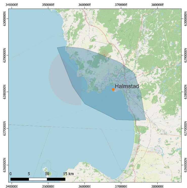
Figur 1. Geografiskt område vid Halmstad specificerat av MSB, samt Sjöfartsverkets mätstation i Halmstad. Bakgrundskarta: OpenStreetMap.
