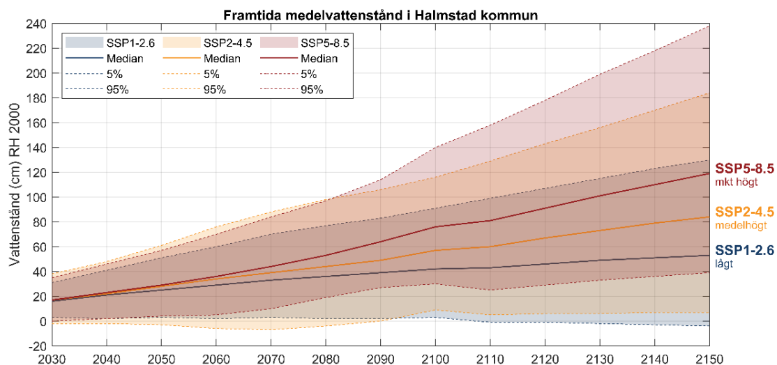
Figur 4. Utveckling av framtida medelvattenstånd i Halmstads kommun under tre olika scenarier, lågt (SSP1-2,6), medelhögt (SSP2-4,5), och mycket högt (SSP5-8,5). Medianvärden visas som heldragna linjer och de skuggade fälten täcker de mycket sannolika intervallen (5:e till 95:e percentil).
