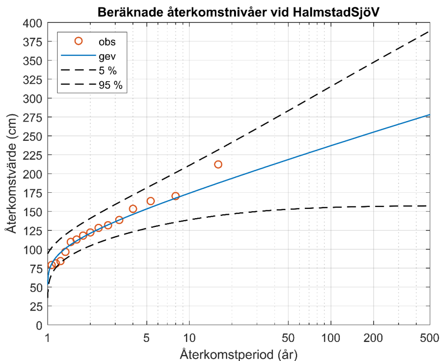
Figur 2. Beräknade återkomstvärden relativt medelvattenståndet vid olika återkomstperioder (blå linje) baserat på årsmaximas från Halmstad (röda cirklar). Streckade linjer (svart) anger tillhörande konfidensintervall på 90 %.
