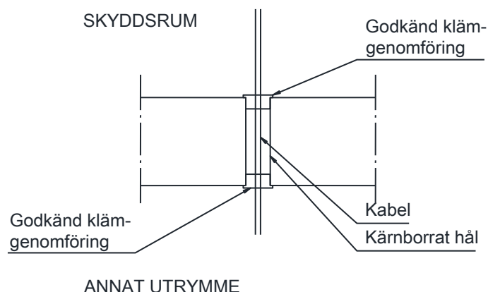
Figur T21-104h. Sektion genom borrarad genomföring med klämgenomföring i golv mot annat utrymme eller skyddsrum.
