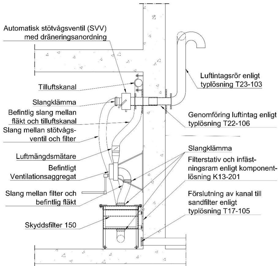
Figur T13-104a. Sektion efter utbyte av sandfilter.
