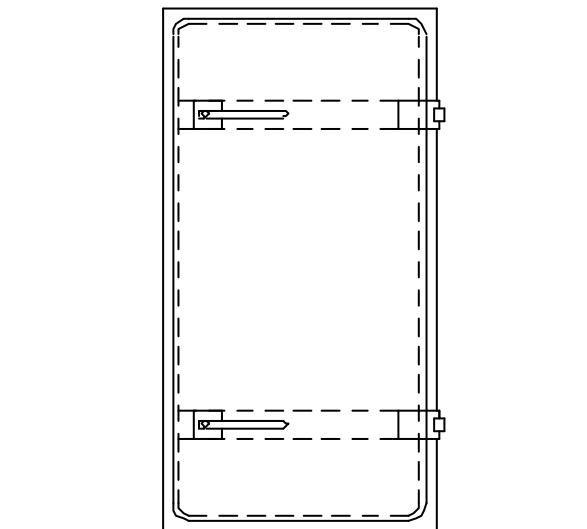
Figur T04-302a. Vy av gastät dörr.
