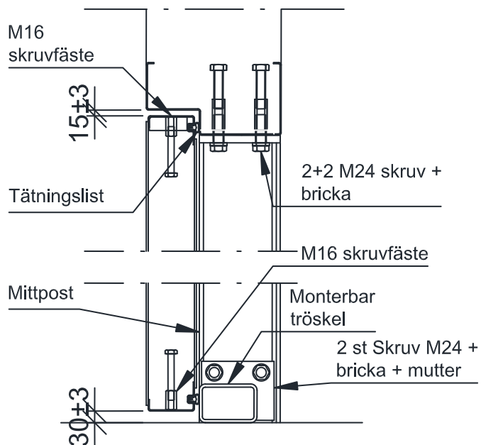
Figur T03-108m. Sektion d monterad dörr.
