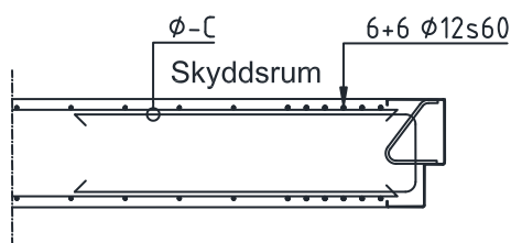
Figur T03-108e. Horisontalsektion på armering vid sidan om karm.
