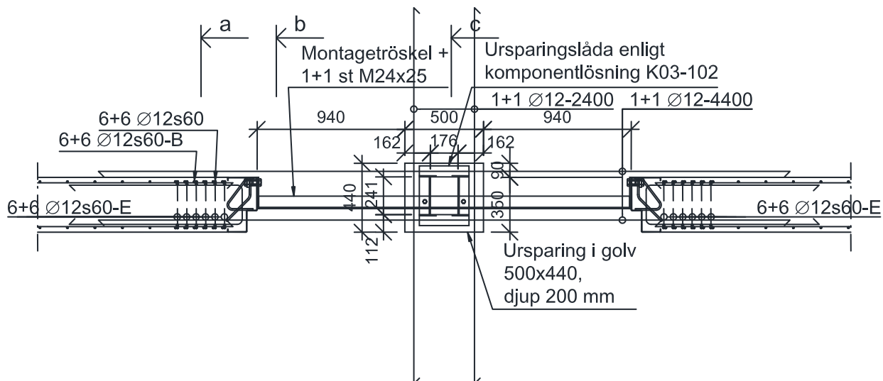
Figur T03-108a. Plan av armering i golvplatta
