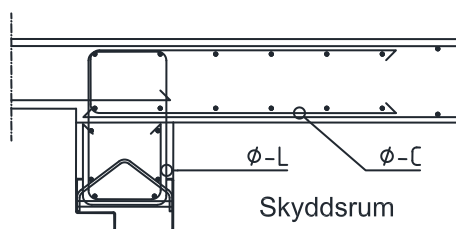
Figur T03-108f. Vertikalsektion på armering ovanför karm.
