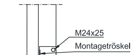
Figur T03-108c. Sektion b av montageträskel.
