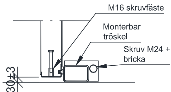
Figur T03-108n. Sektion e monterad dörr.
