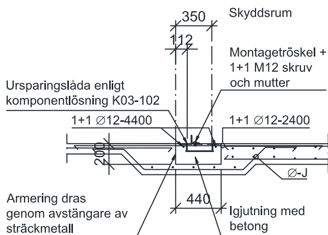
Figur T03-108d. Sektion c av montageträskel.
