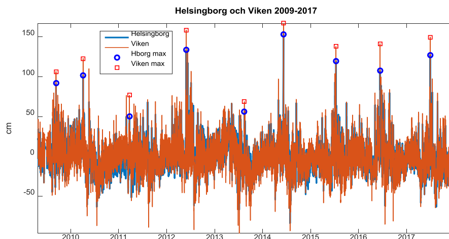
Figur 4. Vattenståndet vid Viken (SMHI) och Helsingborg (Sjöfartsverket) 2009-2017. Vattenståndet anges relativt lokalt medelvattenstånd. Årsmax för de båda stationerna visas som röda kvadrater (Viken) och blå cirklar (Helsingborg).
