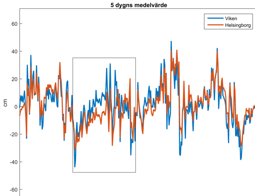
Figur 5. Medelvärde av vattenstånd under 5 dygn. Perioden som visas är vintern 2011. I ramen ser vi att under en period skiljer sig vattenståndet mellan Helsingborg och Viken på ett sätt som avviker från resten av mätserien.
