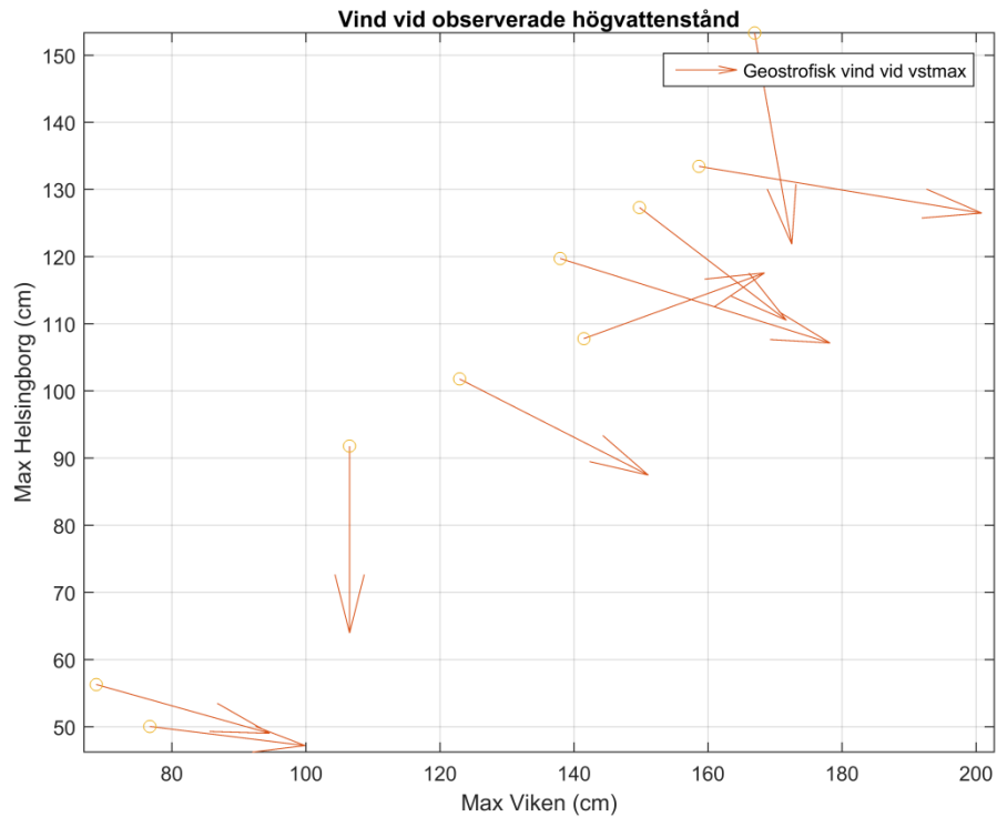
Figur 6. På x-axeln visas årshögsta vattenstånd vid Viken, med samtidigt vattenstånd i Helsingborg på y-axeln, gula ringar. Pilarna visar geostrofisk vind vid samma tid. Pil nedåt = nordlig vind. Pil åt höger = västvind osv.
