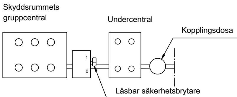
Figur T21-102a. Vy av gruppcentral med säkerhetsbrytare och undercentral.
